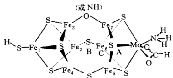
图 1 分子氮与 FeMo-辅基平躺式络合的量化计算模型
